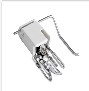
Unité pour double transport avec guide de matelassage
