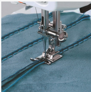
Pied pour pose de cordonnets (H)
