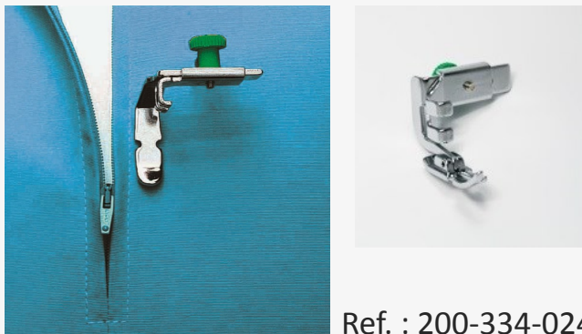
Pied étroit pour pose de fermeture éclair
