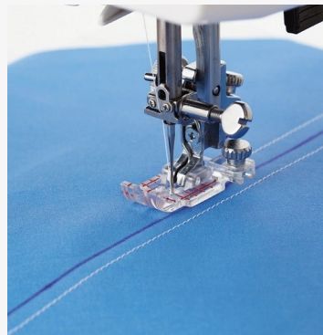
Pied transparent ¼ de pouce pour points droits (OM)
